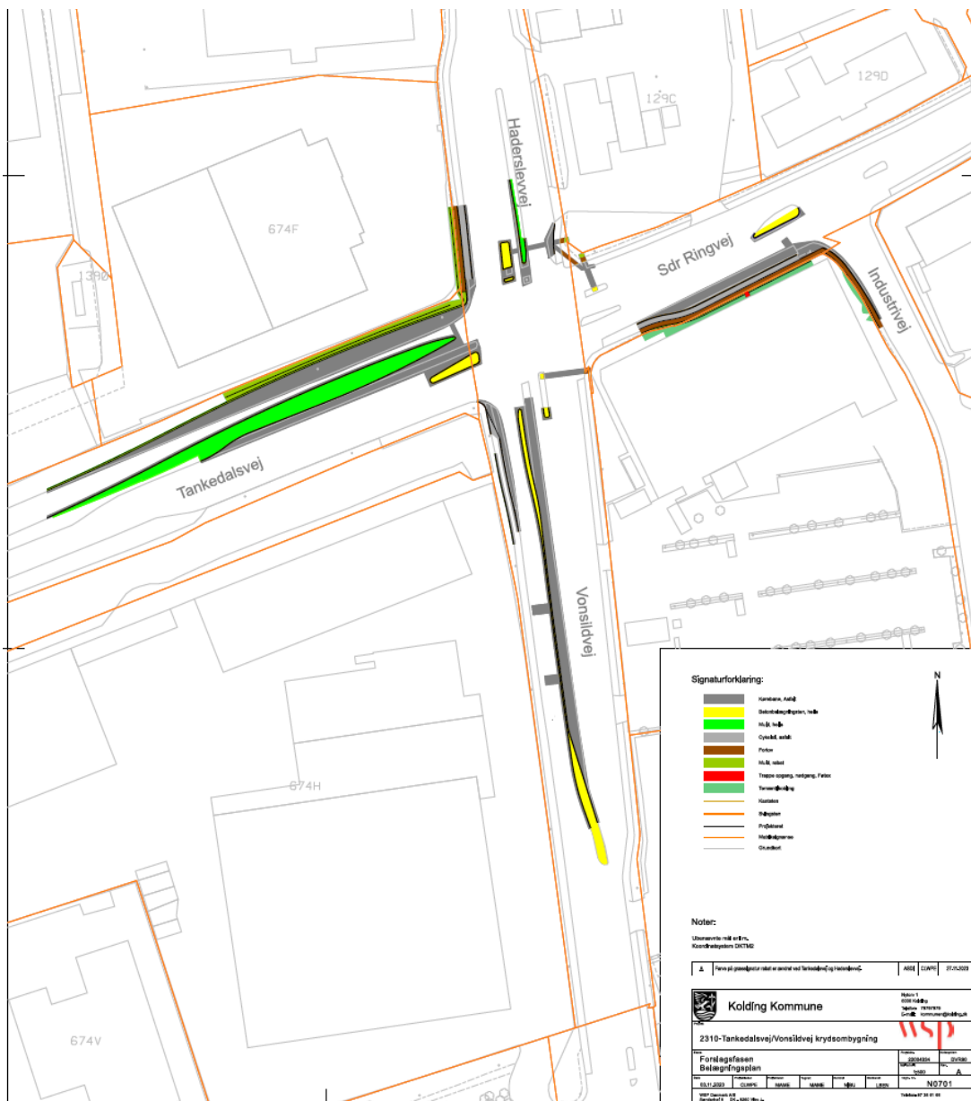
Kort 1. Kortoversigt for projektet: 'Krydsombygning ved Tankedalsvej'.
