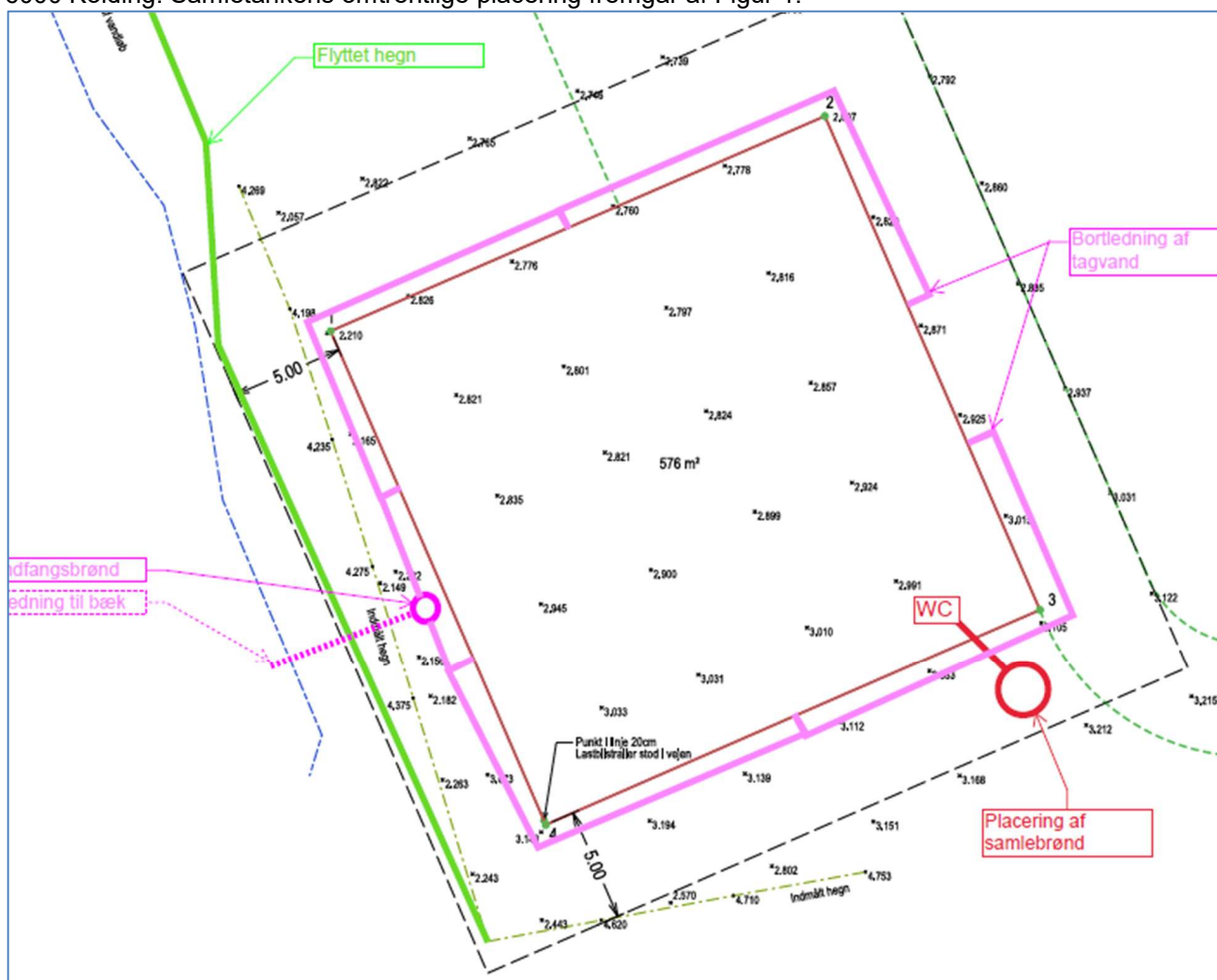
Figur 1: Angivelse af samletank ved transformestation.
