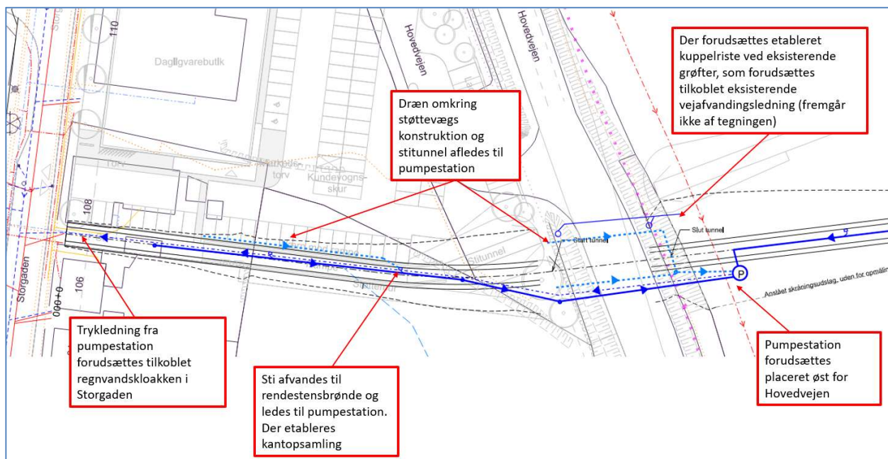
Figur 4: Angivelse af dræn- og regnvandsledninger samt placering af pumpestation.
