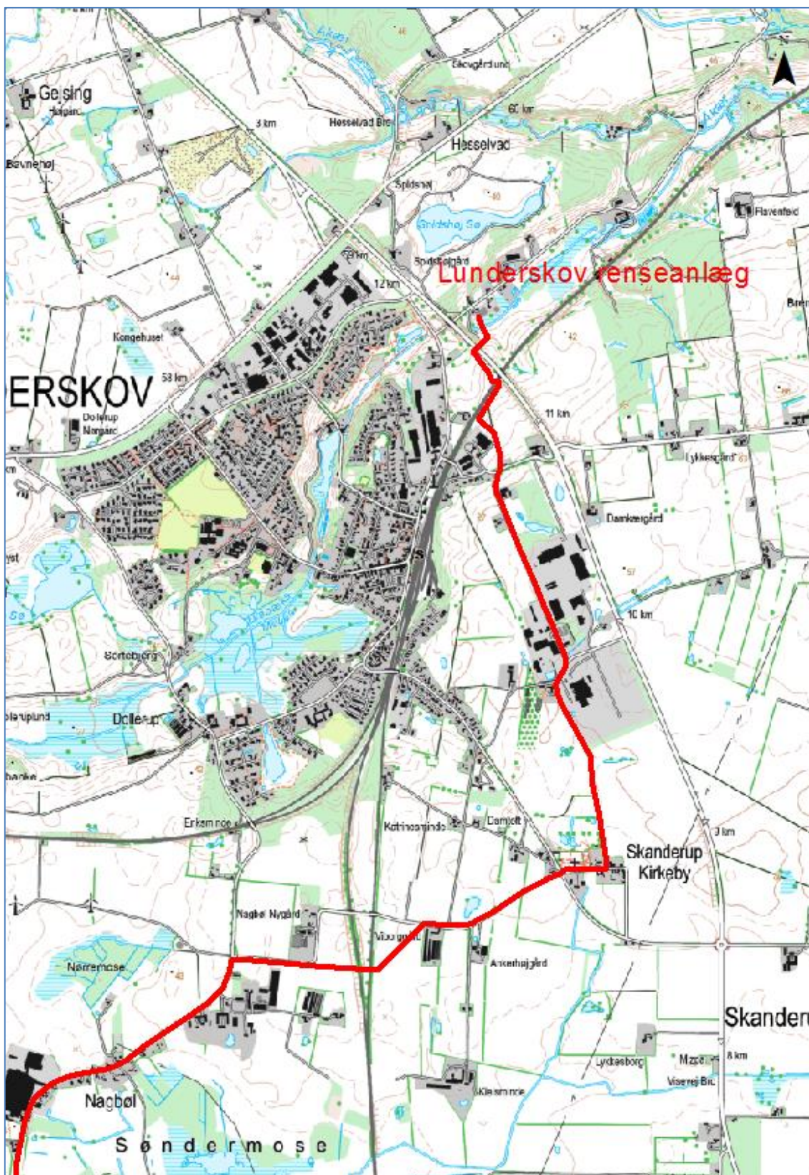
Oversigtskort nord. Nordlige delstrækning af transportledningen fra Lunderskov renselanlæg til Nagbøl.
