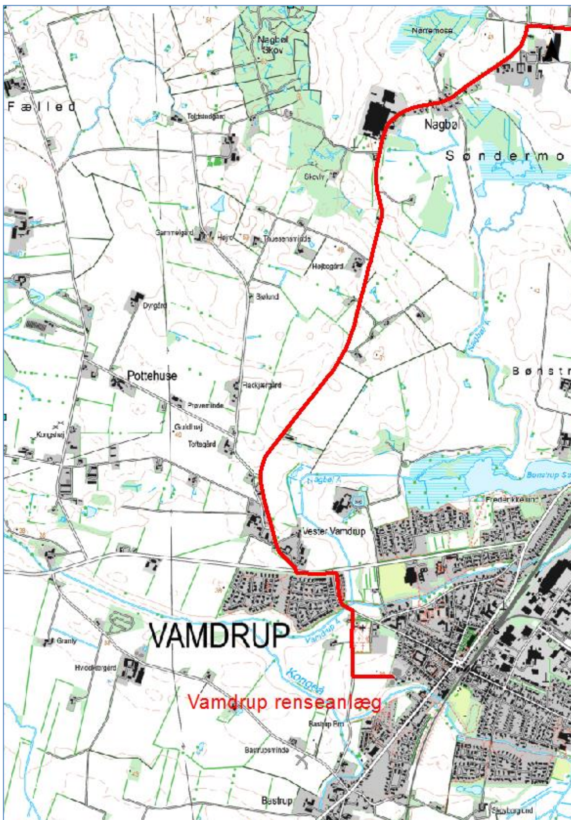
Oversigtskort syd. Sydlige delstrækning af transportledningen fra Nagbøl til Vamdrup renselanlæg.
